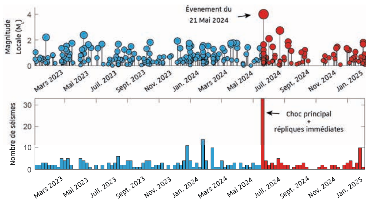
Figure 2-2 Sismicité dans un rayon de 10 km autour de l'épicentre du séisme du 21 mai 2024 enregistrée par le BCSF-Rénass entre janvier 2023 et décembre 2024. En rouge, sismicité enregistrée du 21/05/2024 au 31/12/2024. B. Derode, EOST-ITES, janvier 2025.
