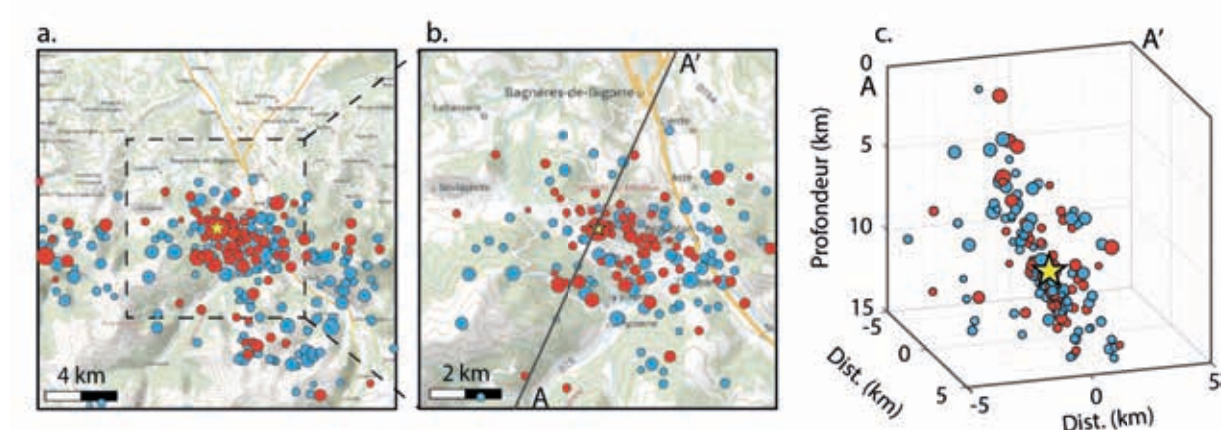
Figure 2-1 Sismicité autour de l'épicentre du séisme du 21 mai 2024 enregistré par le BCSF-Rénass durant la période 2023-2024. En bleu clair les séismes du 01/01/2023 au 21/05/2024, en rouge les séismes du 21/05/2024 au 31/12/2024.
