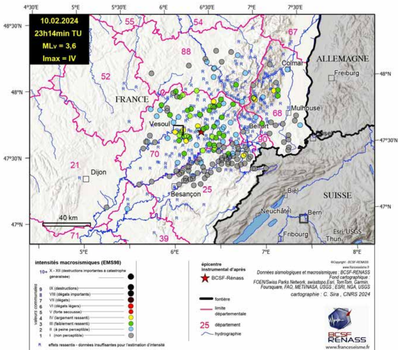
Fig. 2-1 Carte d'intensités macrosismiques
